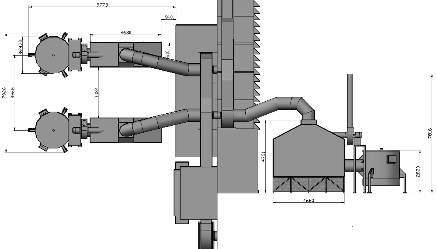
Подключение теплогенераторов ОТД к сушилке ДСП-32. Вариант 1
